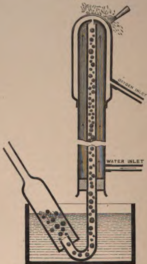
Ozone Apparatus.
